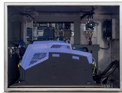
vano quadro elettrico montato su piastra estraibile
